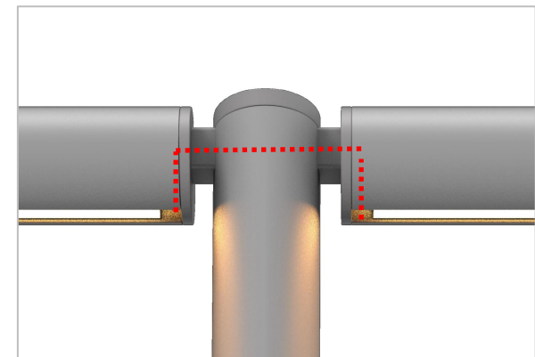
上盖可拆装 (螺纹连接固定) 按图示红色虚线接线 (隐藏式电源线)
